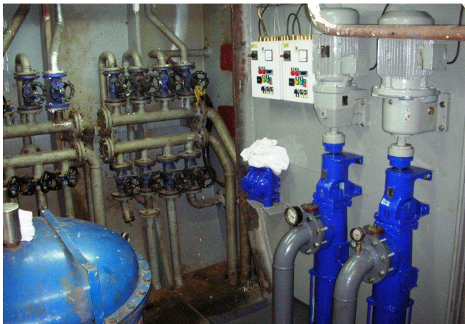
neu überholte Schlamm- und Lenzpumpe
