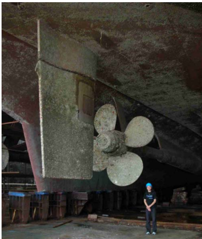
IRIS NEBEN EINER UNSERER SCHIFFSSCHRAUBEN UND DEM RUDER
